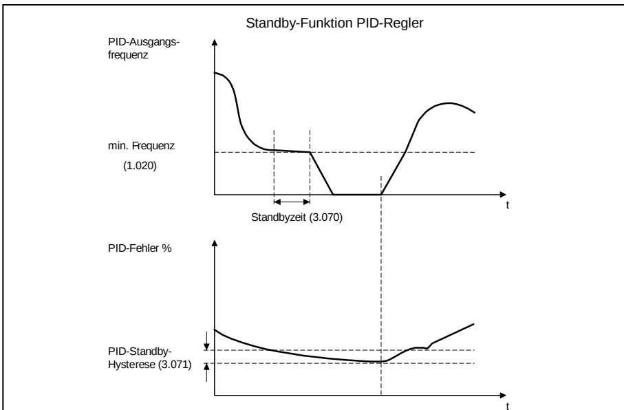
Abb. 41: Standby-Funktion PID-Prozessregelung
