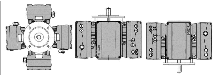
Abb. 10: Motoreinbaulage/ Zulässige Ausrichtungen
