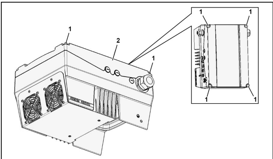
Abb. 34: Demontage Lüfter BG. D
