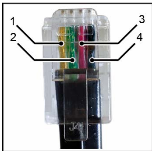
Abb. 9: RJ9 Steckverbinder
