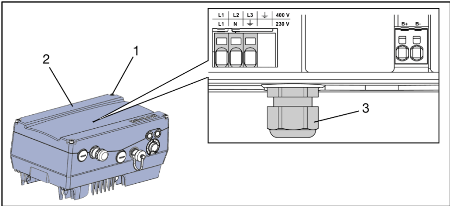
Abb. 16: Leistungsanschluss BG A – C
