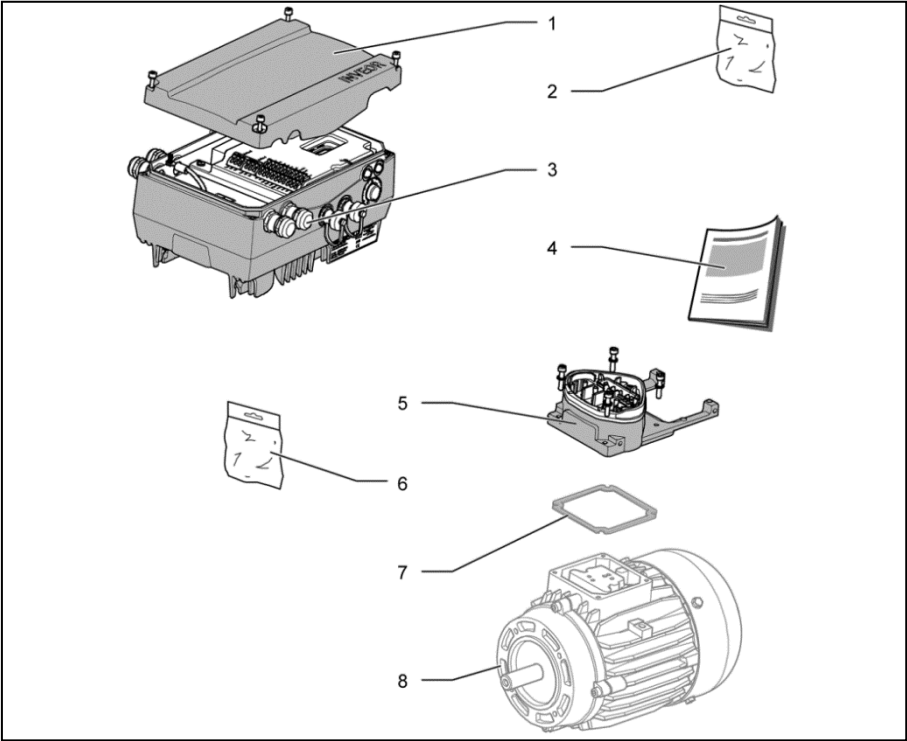
Abb. 7: Lieferumfang
