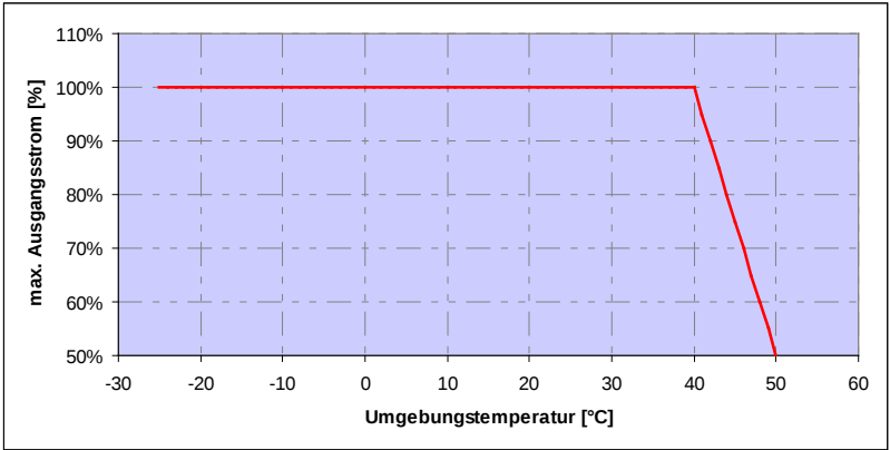
Abb. 44: Derating für wandmontierte Antriebsregler (Baugrößen A – C)
