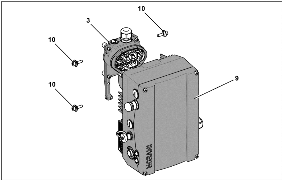
Abb. 25: Antriebsregler aufsetzen
